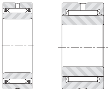
NA Serie 1000, 2000, 22000 NA Serie 3000
