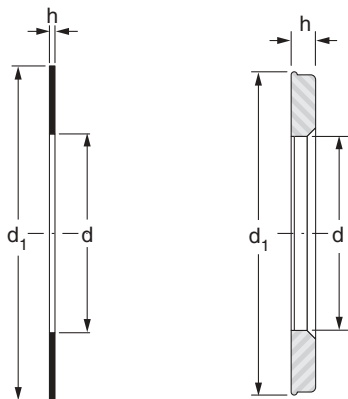
CP dünne Baureihe CP dicke Baureihe
